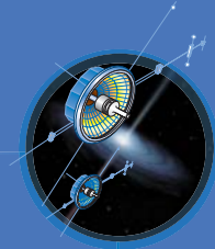
einstein probes
