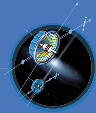
einstein probes
